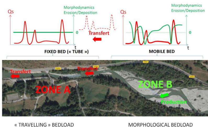
Figure 22: Relation entre morphologie et charriage
