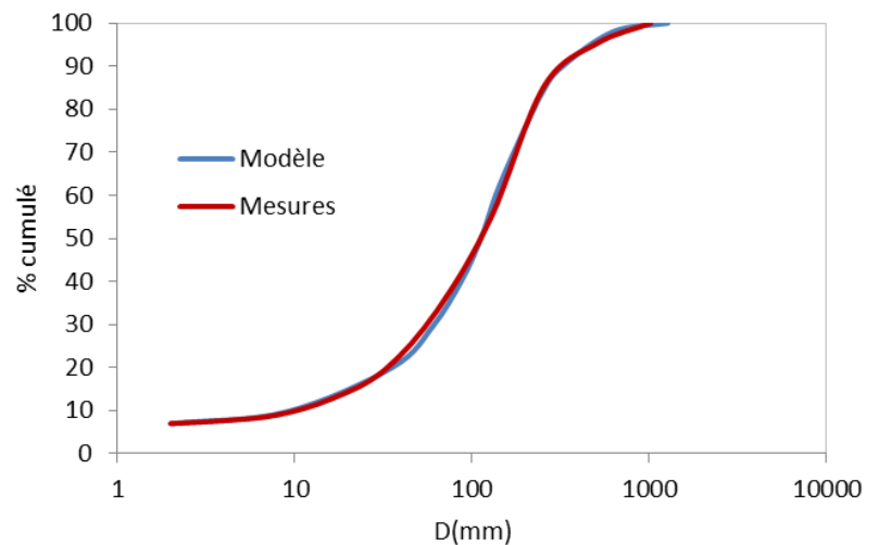
Figure 3: Modélisation de la courbe granulométrique de l'exemple du Tableau 1 avec le modèle en similitude [Recking 2013].
