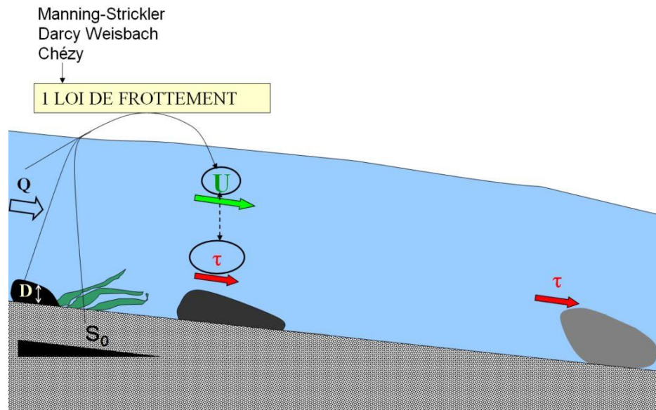
Figure 9: Principe d'utilisation de la loi de frottement
