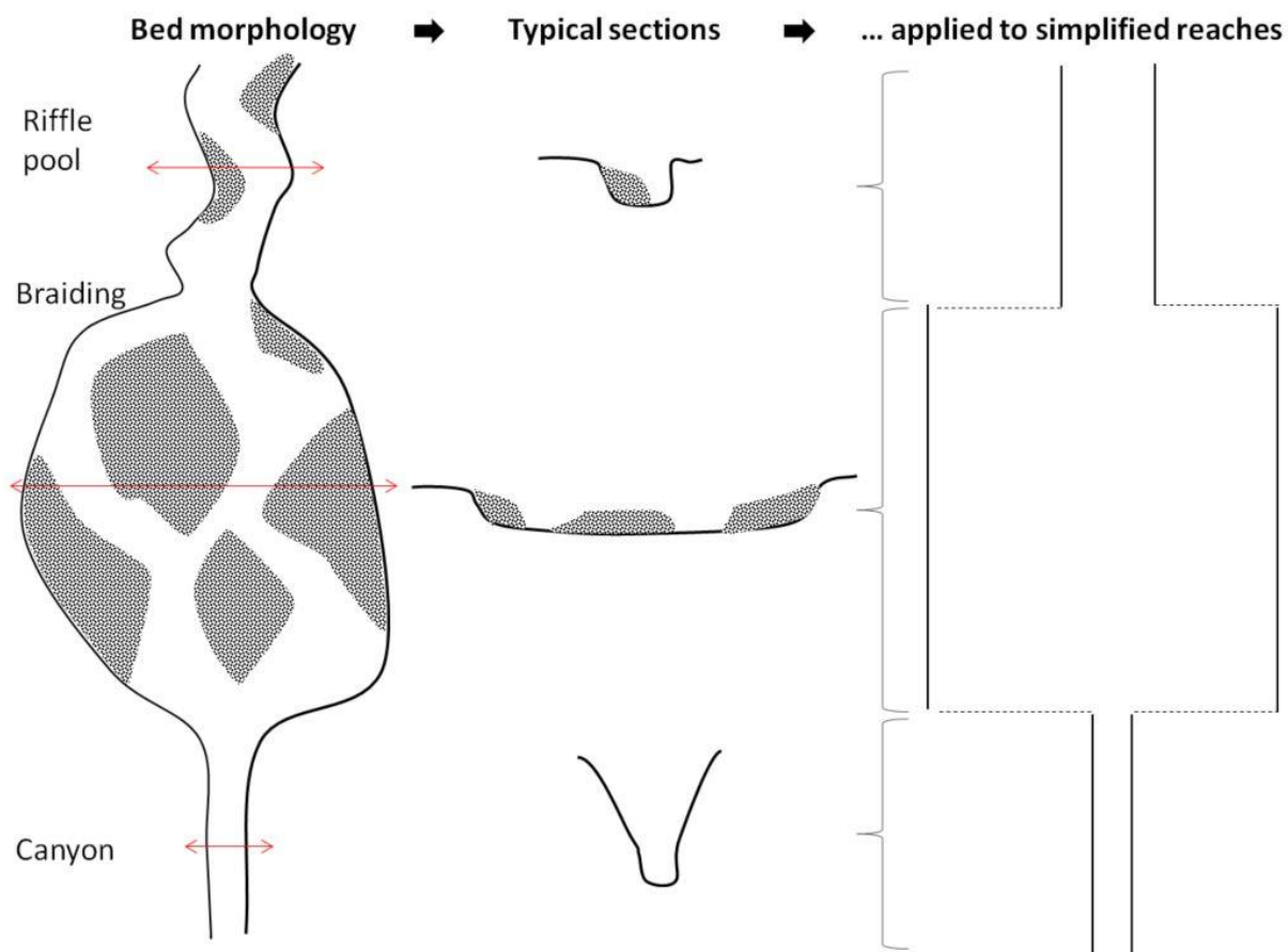
Figure 5: Approximation de la géométrie du lit par une succession de tronçons uniformes
