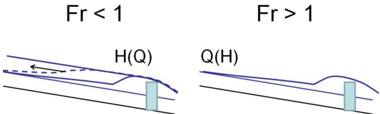
Figure 7: Impacts d'un obstacle introduit dans l'écoulement en fonction du nombre de Fr
