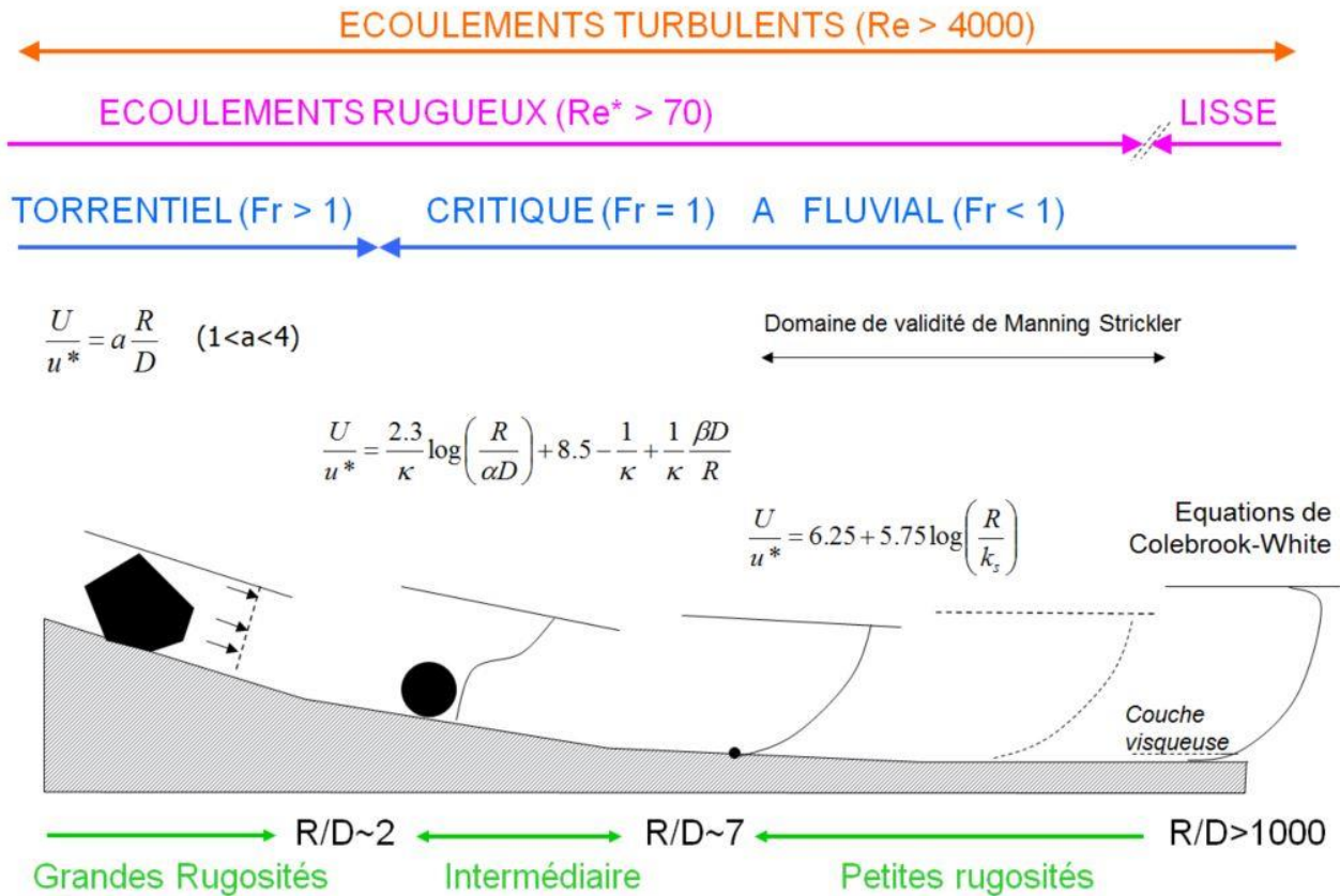
Figure 14: Variation de l'hydraulique avec la pente
