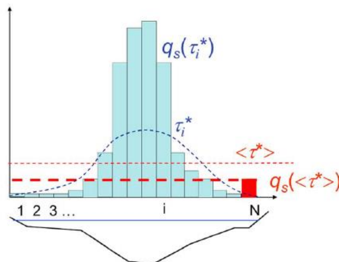
Figure 26: Effets de la variabilité sur la section : le calcul avec une hauteur moyenne ( q_s(\langle \tau^* \rangle) , en rouge) sera inférieur à la somme des calculs locaux ( \sum q_s(\tau_i^*) en bleu) [Recking 2013]
