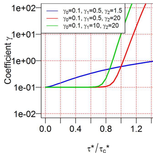
Figure 31: Variation du coefficient gamma (i.e., de la mobilité au sein d'une classe donnée) avec le taux de transport.
