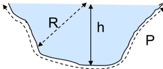
Figure 6: Représentation schématique du rayon hydraulique
