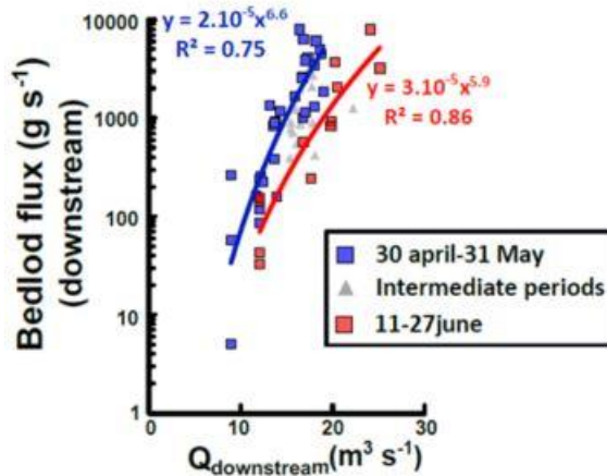
Figure 25: Variabilité saisonnière du charriage sur la Séveraise [Misset et al. sub]
