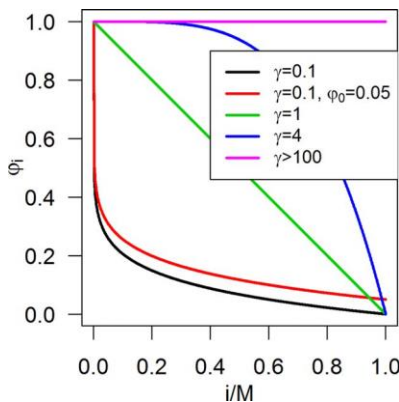
Figure 30: Fraction \varphi_i du i^{\text{th}} percentile de la granulométrie de surface ( i[0,M] ) qui est mobile pour la contrainte hydraulique appliquée.
