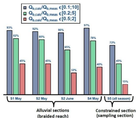
Figure 23: Comparaison du charriage mesuré avec des calculs réalisés en plusieurs sections de la rivière Séveraisse [Misset et al. 2020]
