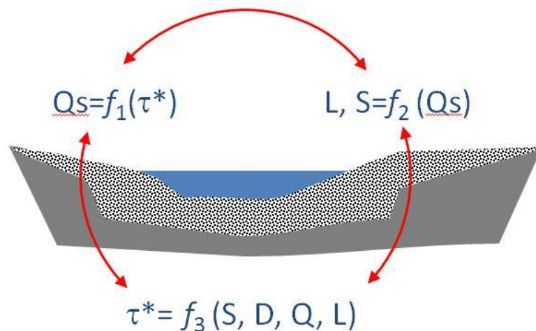
Figure 21: Principe de rétroaction existant entre l'hydraulique, le transport et la géométrie
