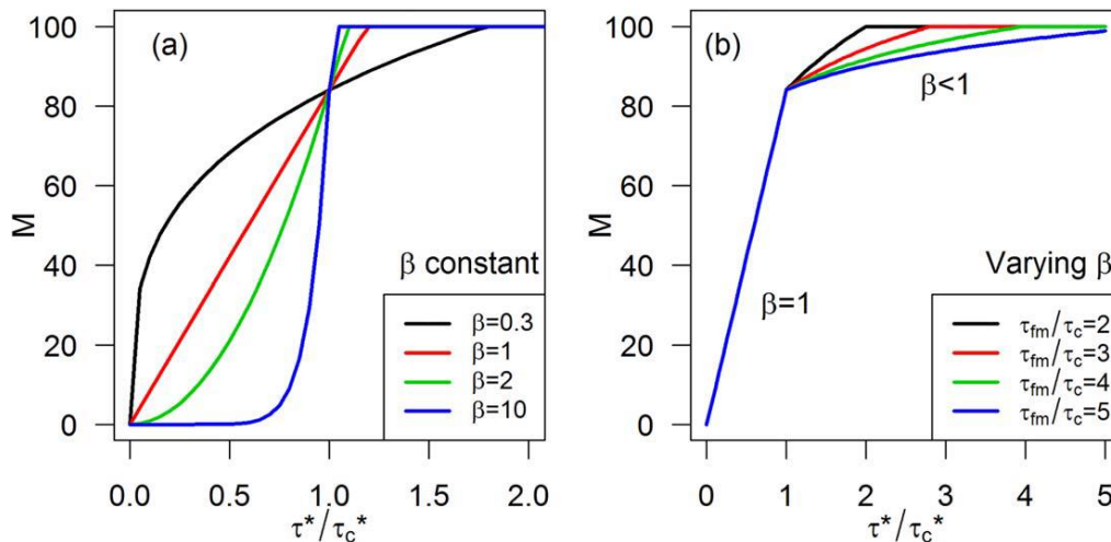
Figure 29: Variation du percentile de taille maximum transportée M avec \tau^* / \tau_c^* , pour Ref=84 , (a) avec \beta constant et (b) avec distinction entre les conditions de transport faibles ( \beta=1 dans l'exemple) et fortes
