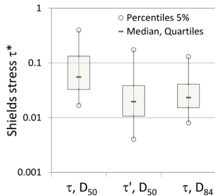
Figure 15: Nombres de Shields calculés pour une large base de données (> 10000 valeurs) a) sans correction de contrainte et avec D_{50} b) avec la correction de MPM et D_{50} c) sans correction de contrainte et avec D_{84}
