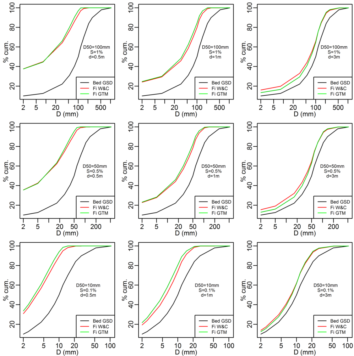
Figure 32: Reproduction des résultats du modèle de Wilcock and Crowe avec GTM pour différentes conditions de transport
